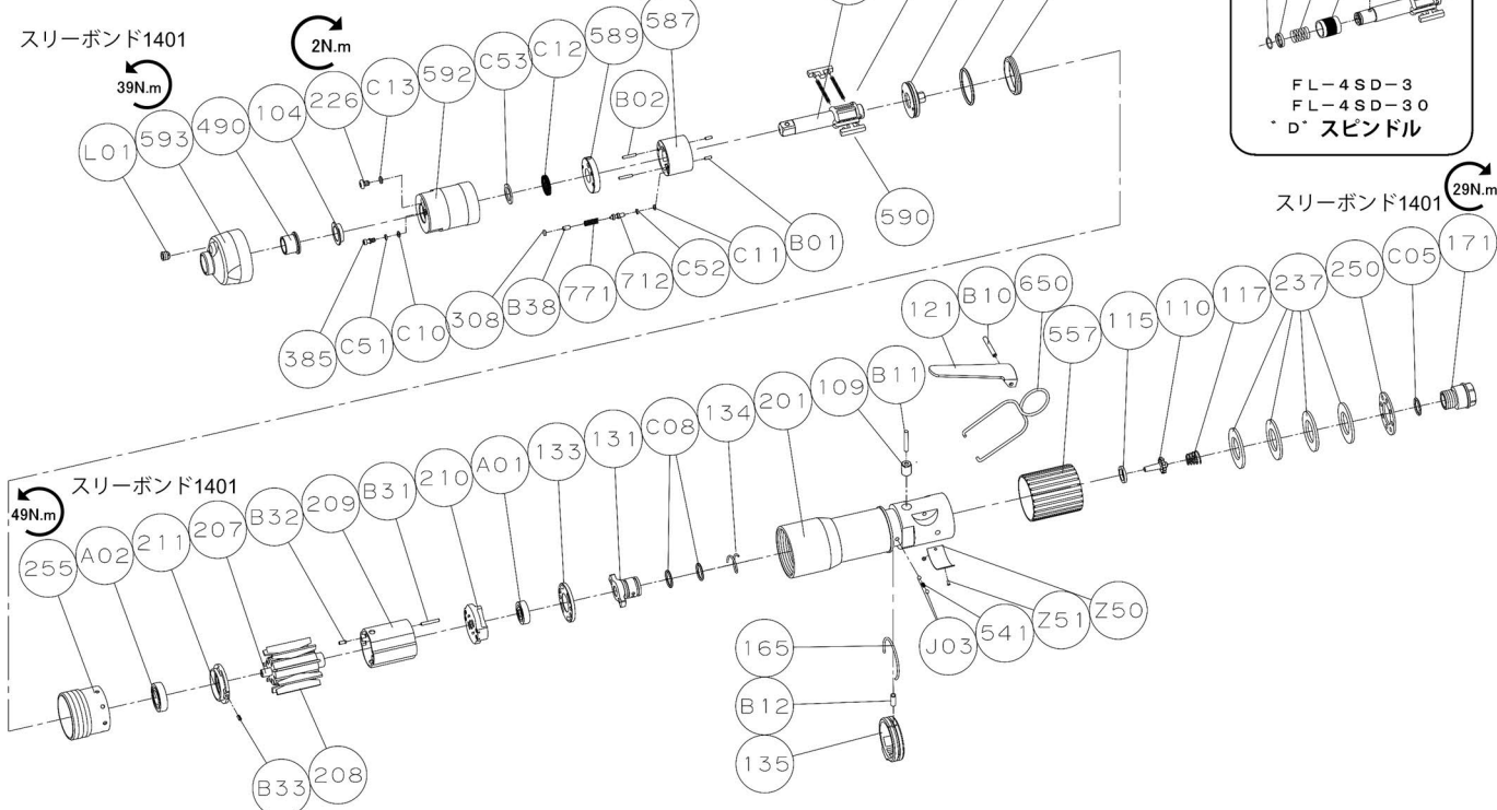
FL-4S-3, -4SD-3, -30
