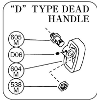
OPTIONAL PART
